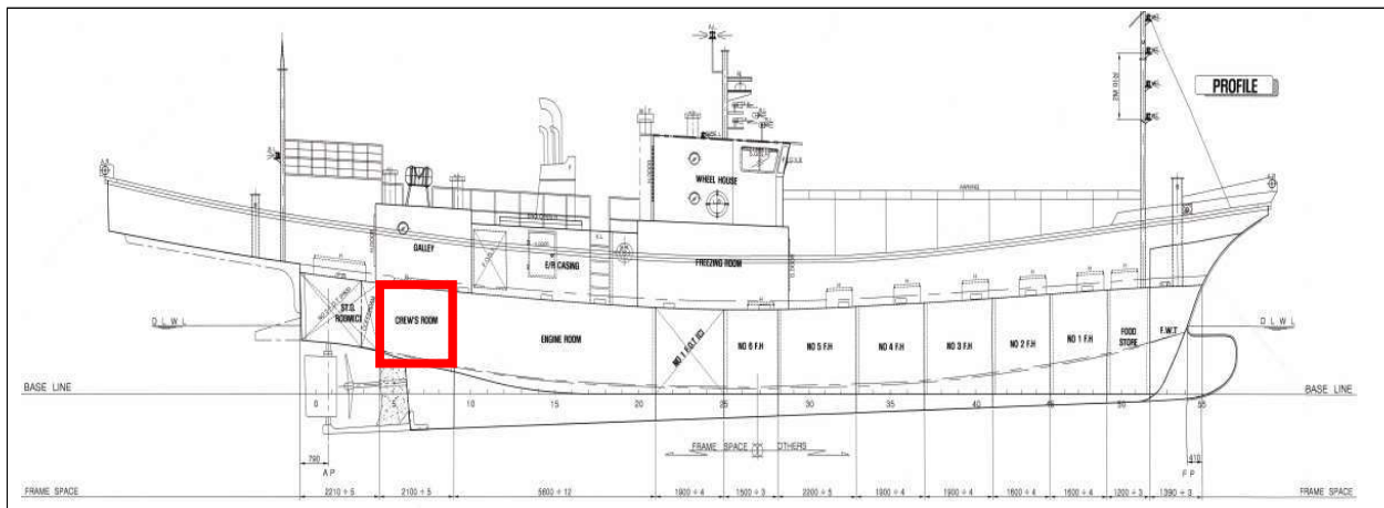
선박 일반배치도(선원실)
